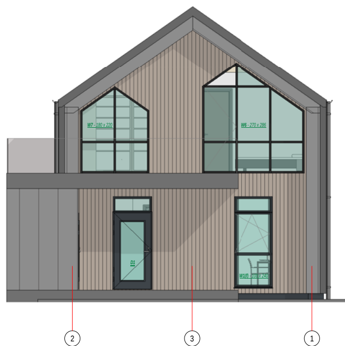
E6 SØR M 1 : 100
