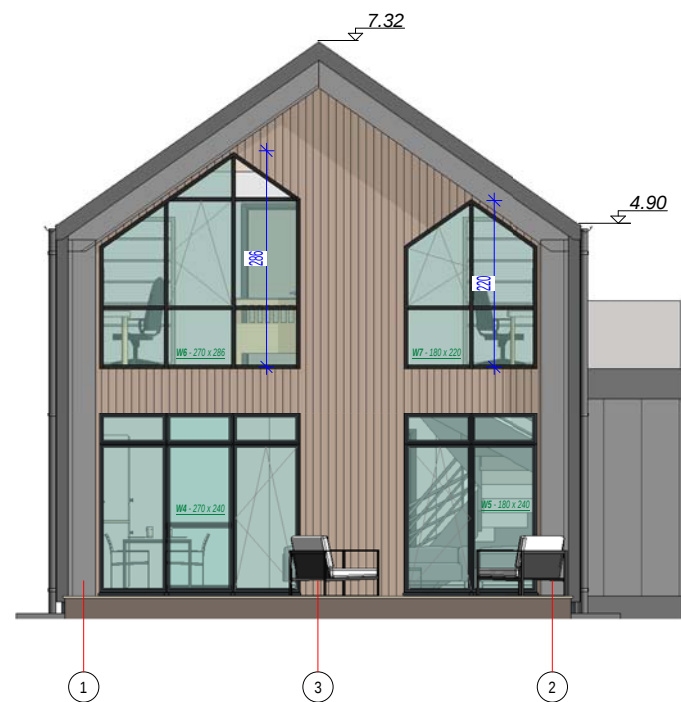
E4 NORD M 1 : 100
