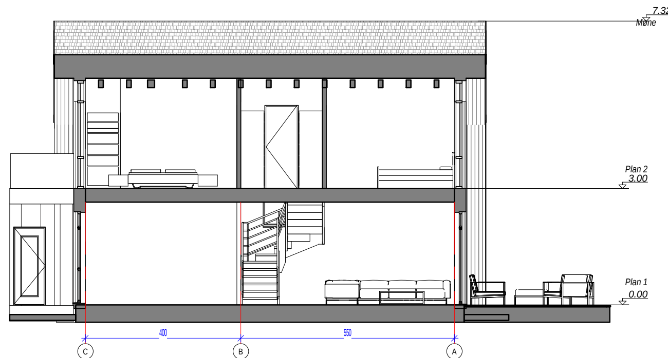
E9 - Snitt 2-2 M 1 : 100
