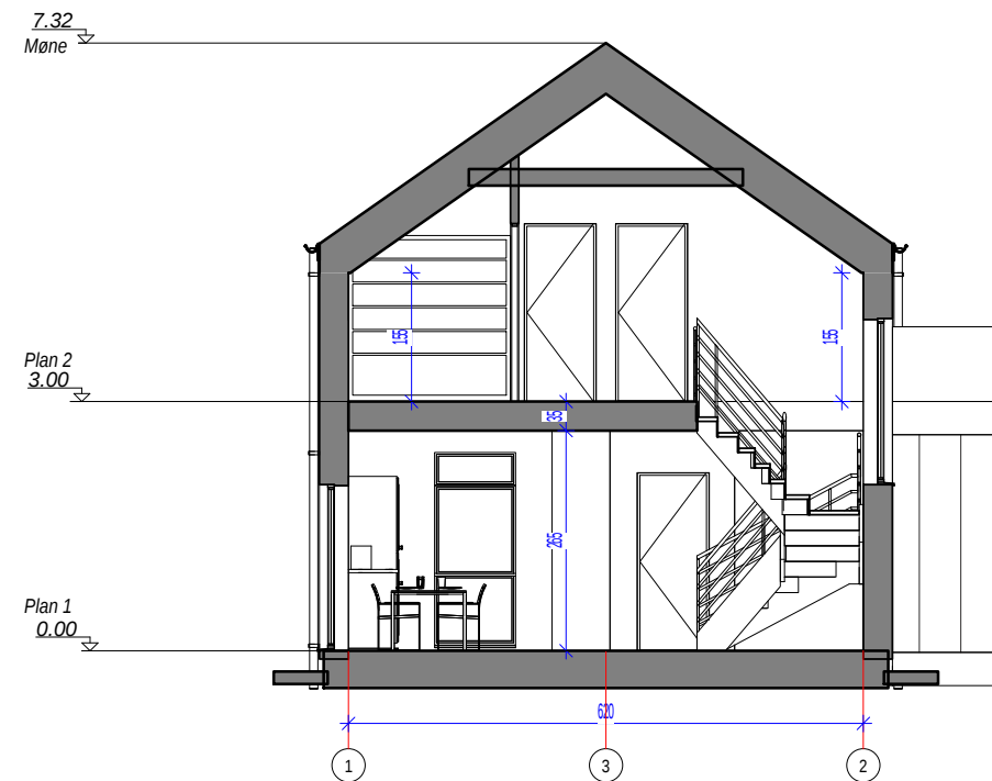
E8 - Snitt 1-1 M 1 : 100
