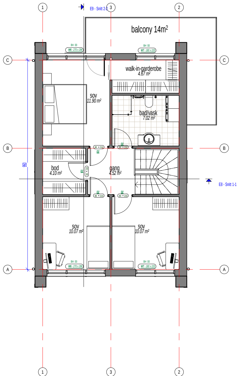
E2 - Andre etasje M 1 : 100
